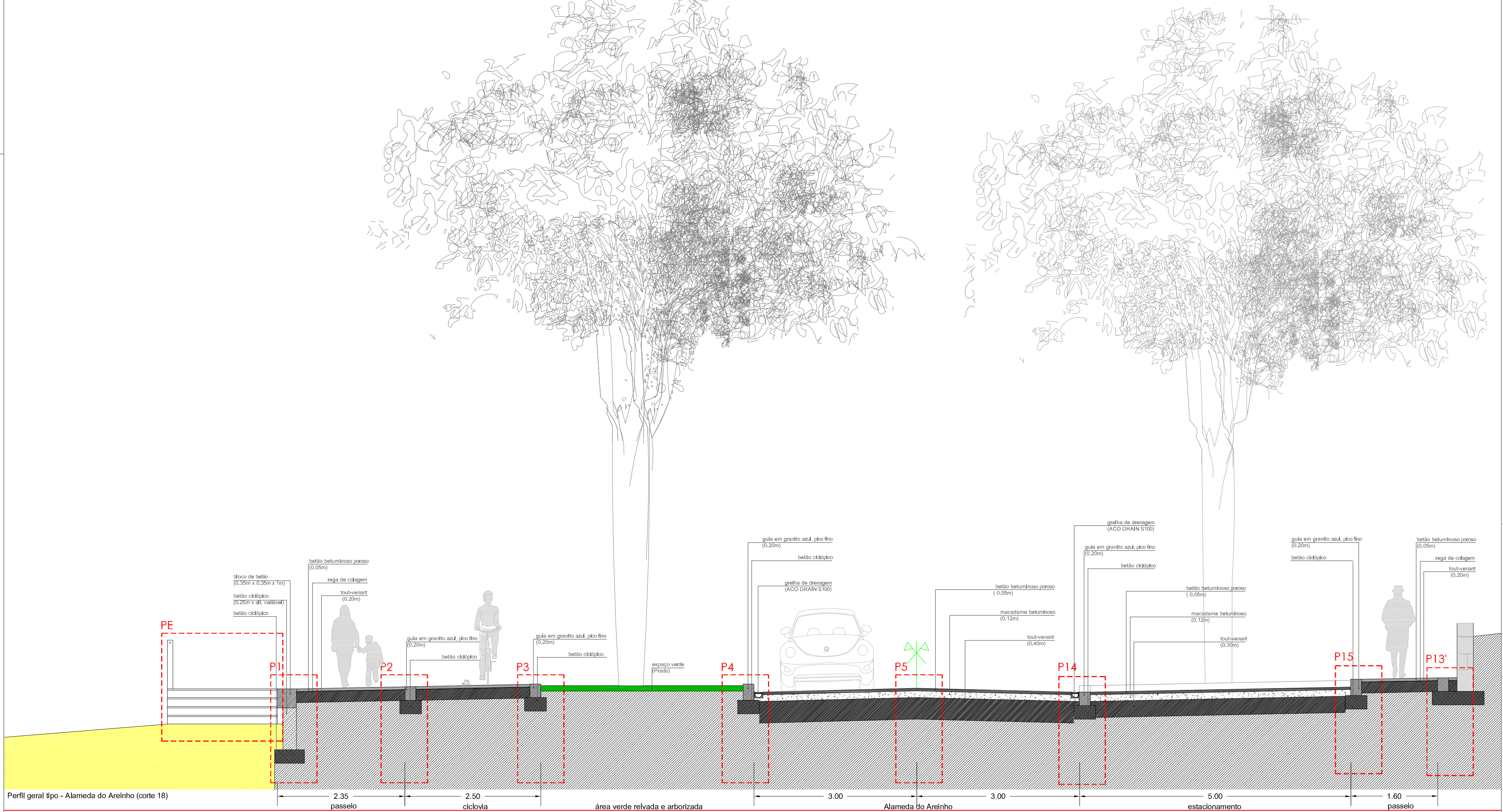
Perfil geral tipo - Alameda do Areinho (corte 16)
